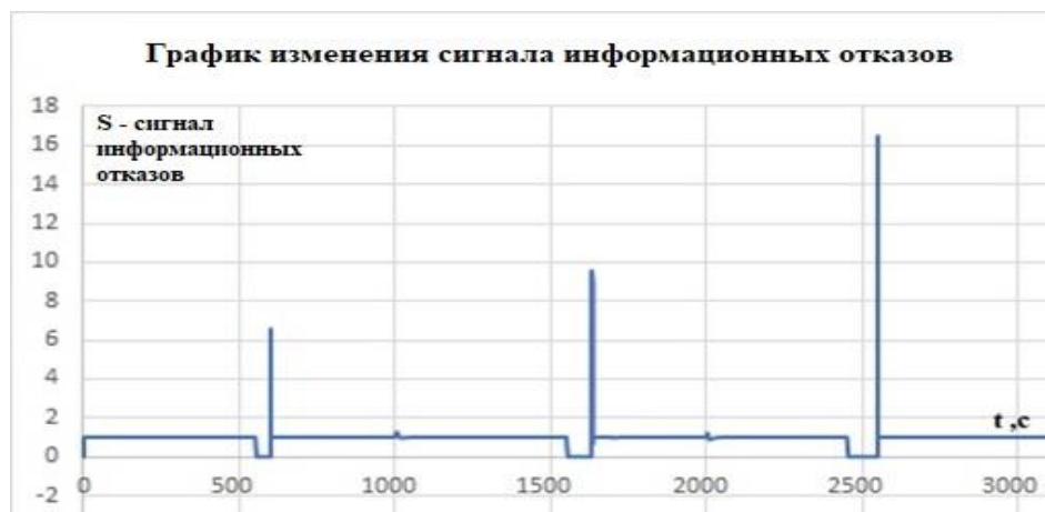
Рисунок 3.29. - График изменения сигнала информационных отказов
