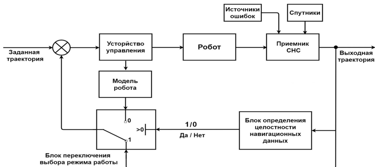
Рисунок 4.1. - Структурная схема системы управления мобильным роботом с выбором режима управления
