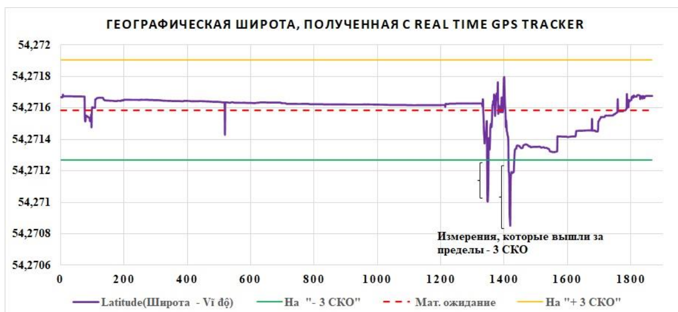
Рисунок 3.13. - Результаты измерения широты в точке 54,27 град. широты и 48,30 град. долготы
