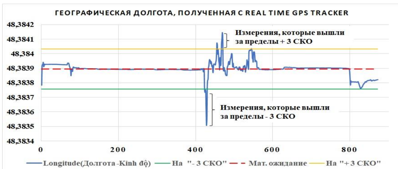
Рисунок 3.10. - Результаты измерения долготы в т. 54,35 град. широты и 48,38 град. долготы
