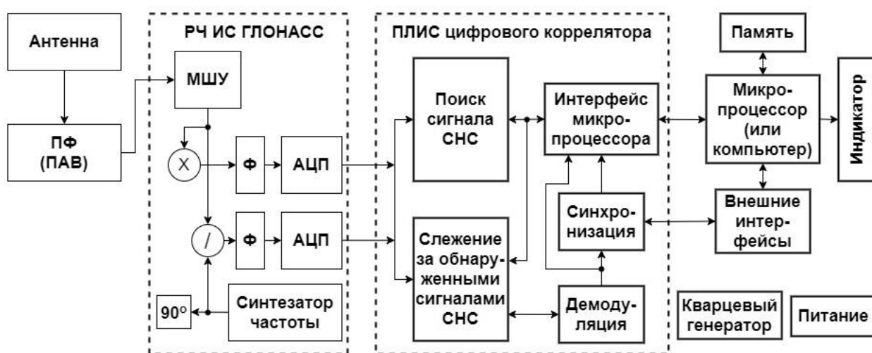
Рисунок 1.2. - Обобщенная структурная схема приемника СНС (на примере ГЛОНАСС)
