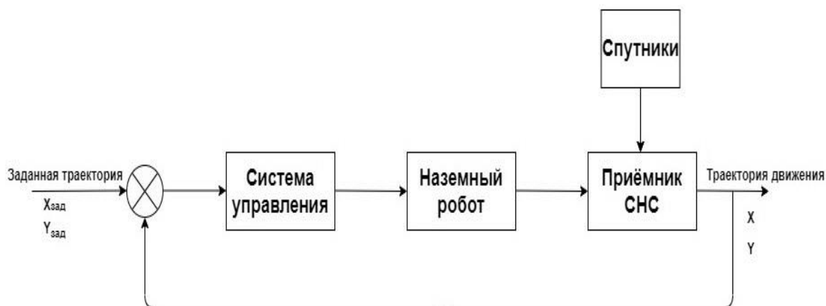
Рисунок 1.1. - Схема управления наземным роботом с СНС
