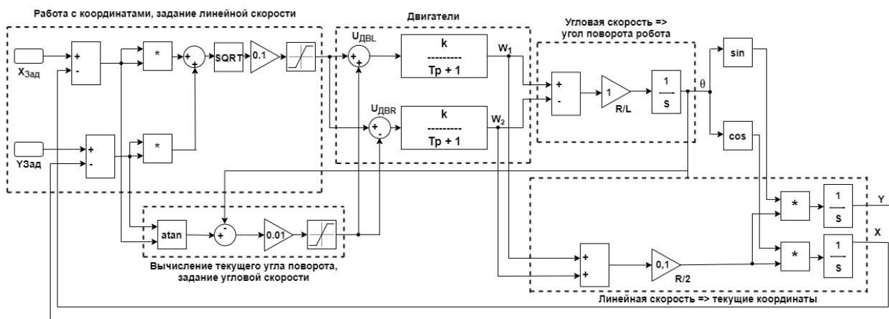
Рисунок 2.6. - Динамическая модель мобильного наземного робота [52].
